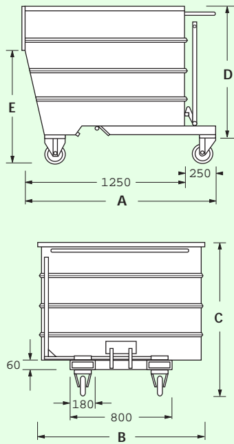
Scatole di inforcazione Fork jackets
