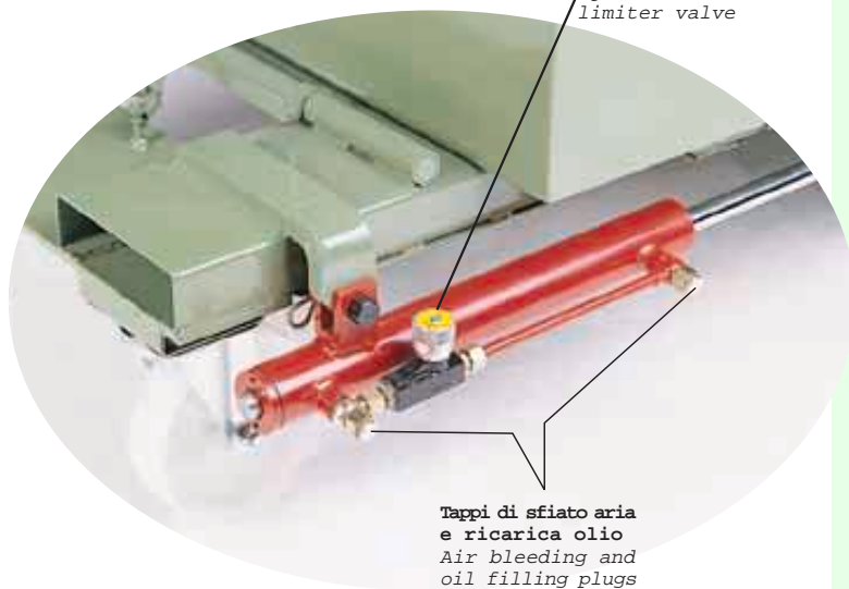
Valvola regolabile limitatrice di flusso Adjustable flow limiter valve
